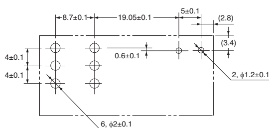
端子排列/内部连接 (顶视图)
